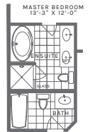
OPTIONAL ENSUITE PLAN
