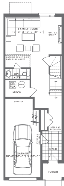
OPTIONAL BATH PLAN
